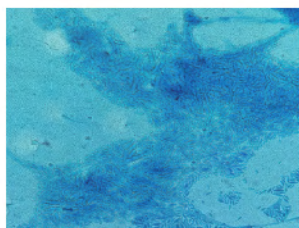
▲棉酚兰染色
