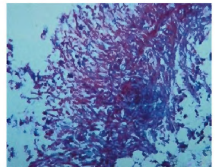
▲镰刀菌孢子
